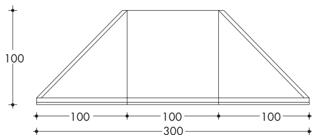
PIANTA
