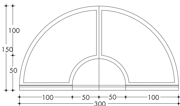
PIANTA
